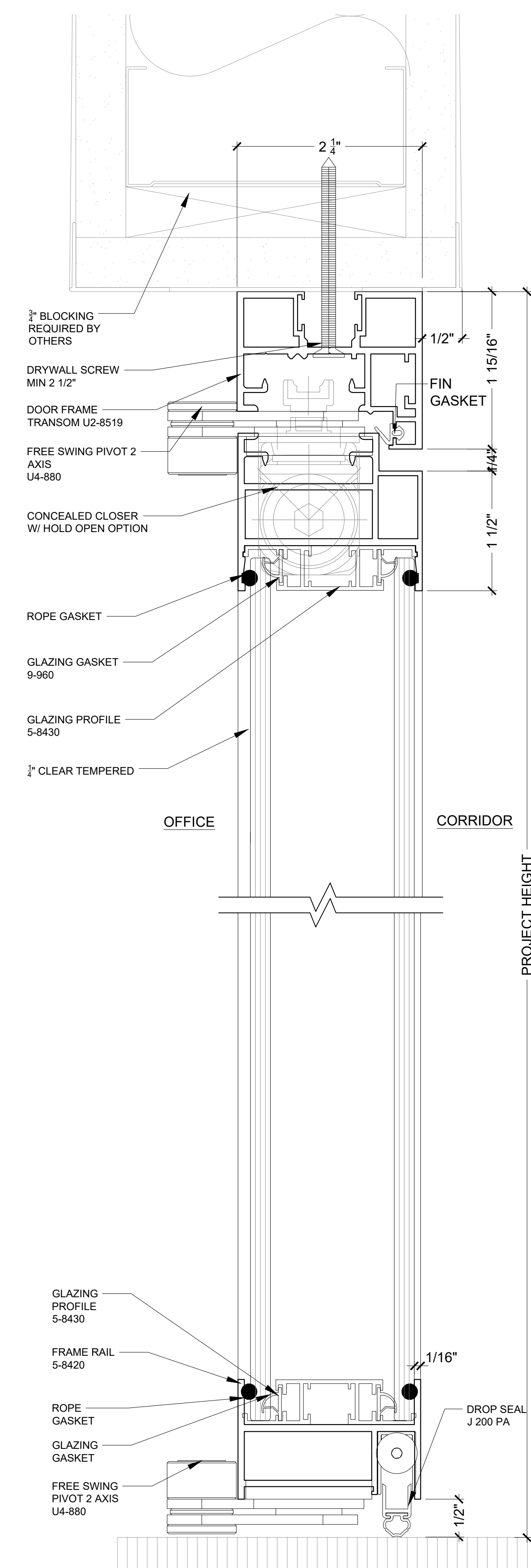
1 FRAMED PIVOT DOOR 1'-0"=1'-0"
